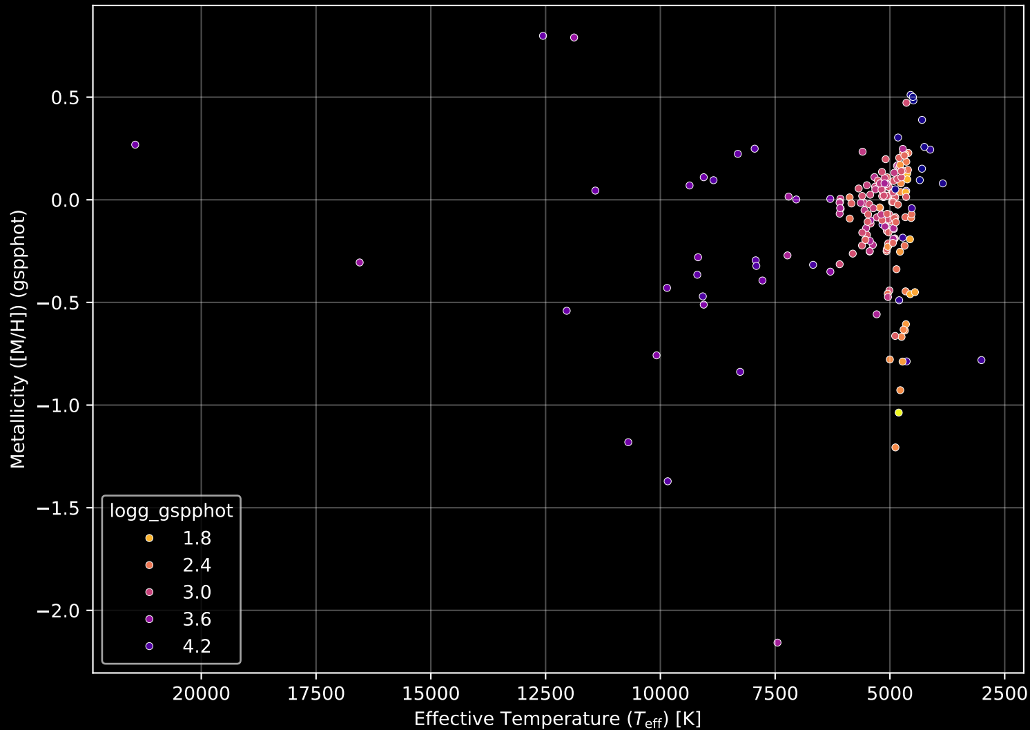
APOGEE DR17 Field: [105+12] Stellar Population Parameters (n= 194)
